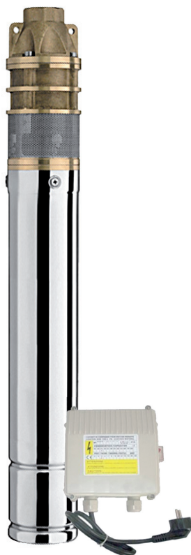
4. BRUNNEN-STAR 750-4 , Impellerpumpe (5 007 006 006)
